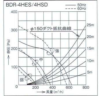
静圧・風量曲線
