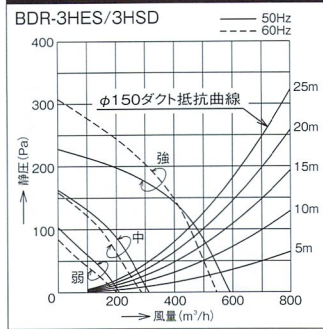
静圧・風量曲線
